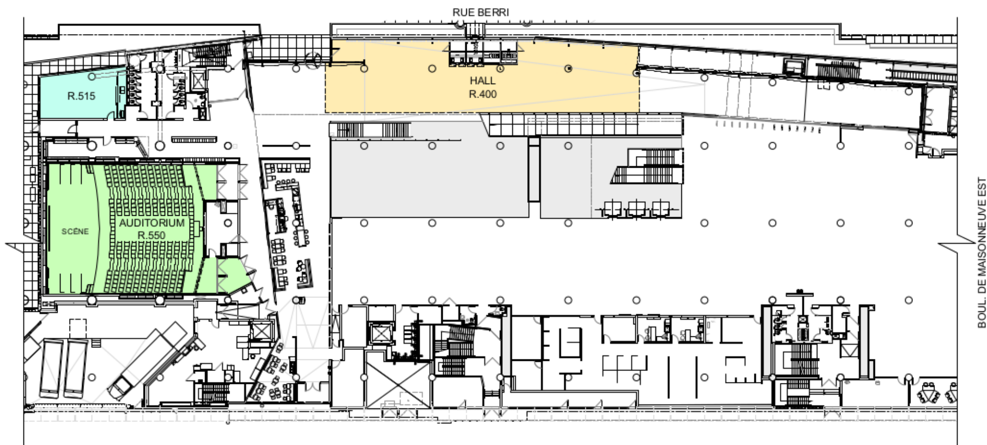
PLAN CLEF NIVEAU RDC ÉCHELLE: 1:500
